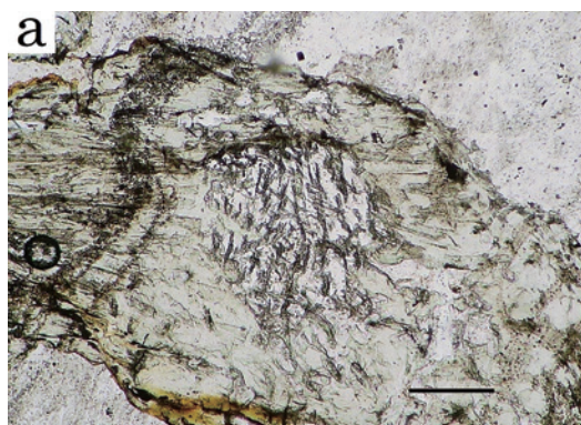
⑥堇青石（crd）花崗閃緑岩に含まれ，花弁状の三連双晶を示す スケール 0.2 mm （本文37－42，保科・関東山地研究グループ）
